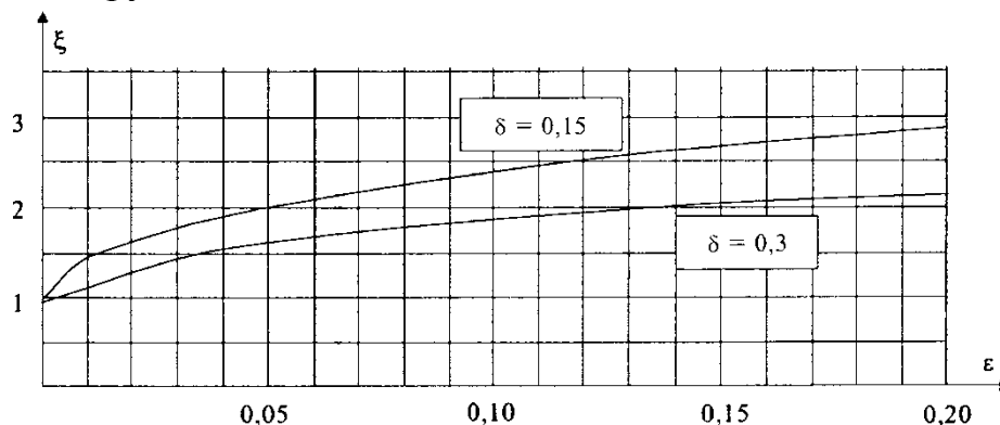
Рисунок 10.1 – Коэффициенты динамичности
