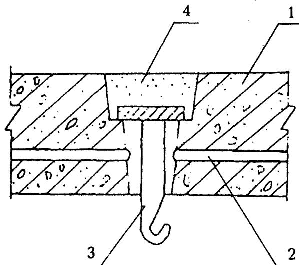
1 — панель перекрытия; 2 — электроканал; 3 — крюк (приварен к круглой стальной пластине); 4 — раствор (заделка нижней части отверстия условно не показана)
