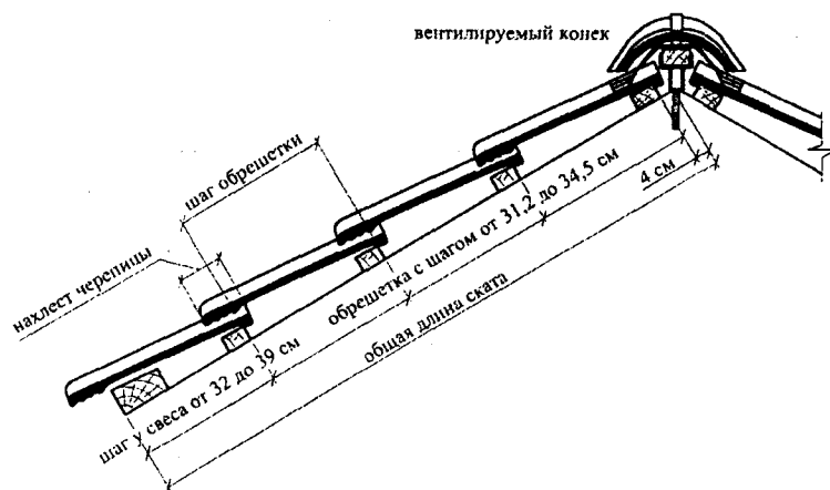
Рисунок К.1 – Поперечный разрез черепичной кровли
