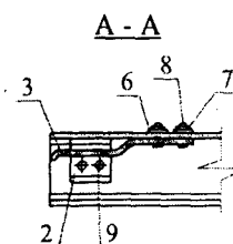
Рисунок Н.2 – Ендова кровли
