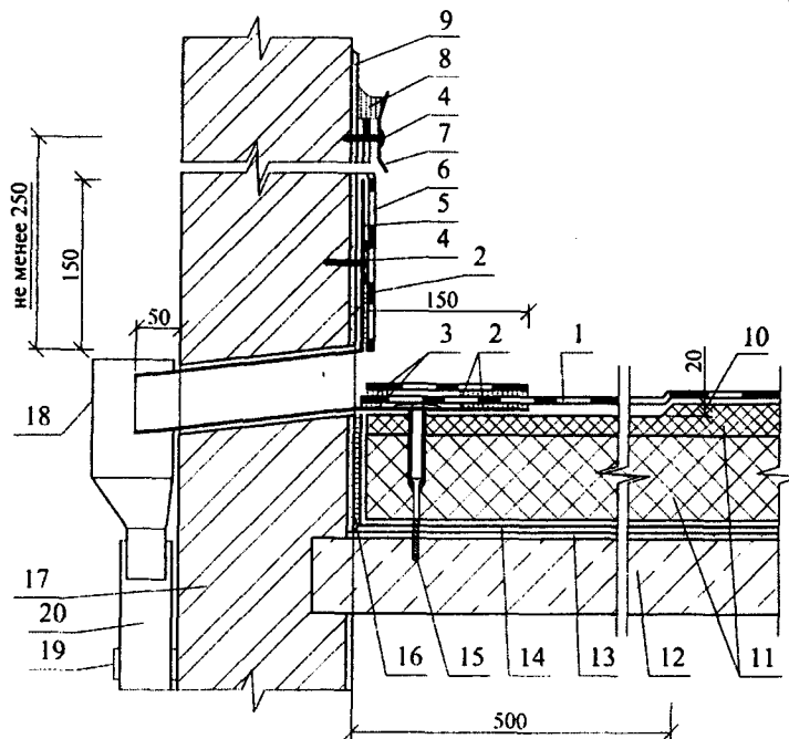
Рисунок Ж.10 – Примыкание кровли к сливу через парапет
