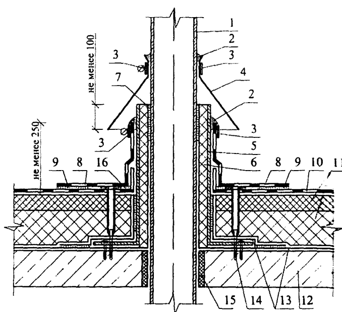
Рисунок Ж.6 – Примыкание кровли к зенитному фонарю
