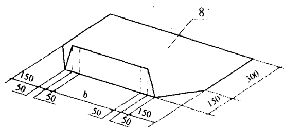
Уголок со стороны конька (b - ширина трубы)
