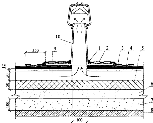
Рисунок В.5 – Пример установки кровельного аэратора (вентиляционного патрубка) над каналом 100 мм
