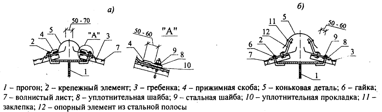
Рисунок Н.7 – Конек кровли глухой (а); вентилируемый (б)
