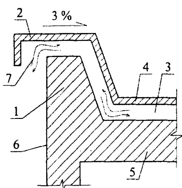
Рисунок В.3 – Схема устройства парапетного узла вентилируемого покрытия
