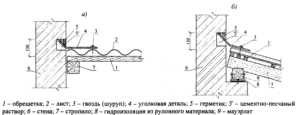
Рисунок Н.6 – Примыкание кровли из волнистых листов к поперечной (а) и продольной (б) стене
